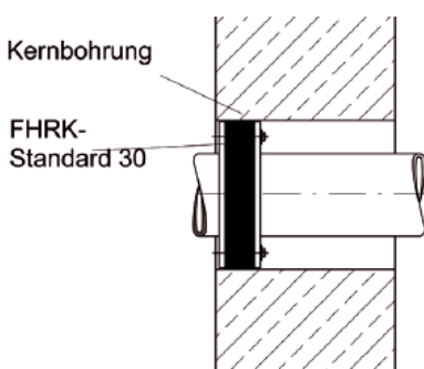
Wandeführung wasserundurchlässige Betonwand mit Kernbohrung
